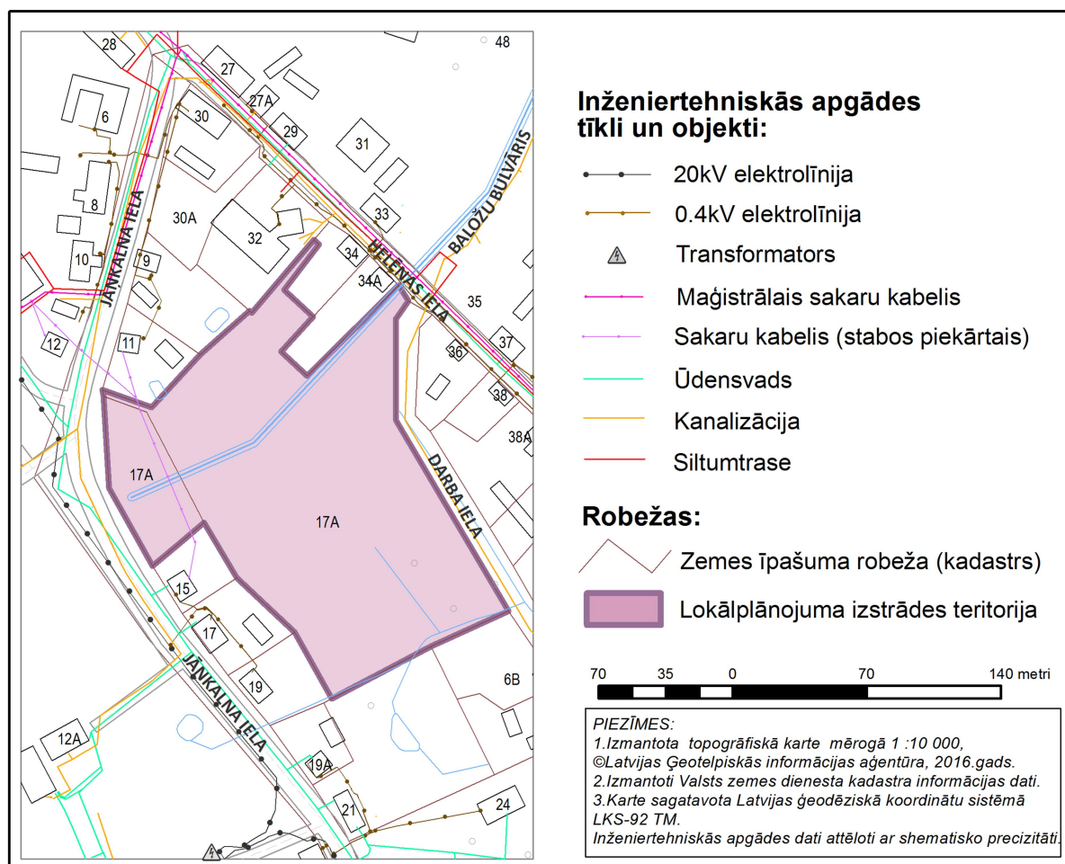
Attēls Nr. 7. Inženierkomunikāciju tīkls gar lokālplānojuma teritoriju.
