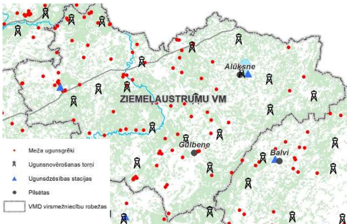
2.7.1. attēls. Meža uguns novērošanas torņu un meža ugunsdzēsības staciju tīkls, kā arī meža ugunsgrēku statistika no 2013.-2018. gadam 11
