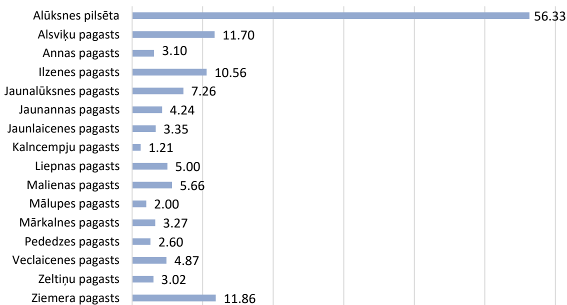
Attēls 9.2. Ūdensvadu tīklu garumi (km) Alūksnes novadā 2021. gadā, Avots: SIA "Rūpe"
