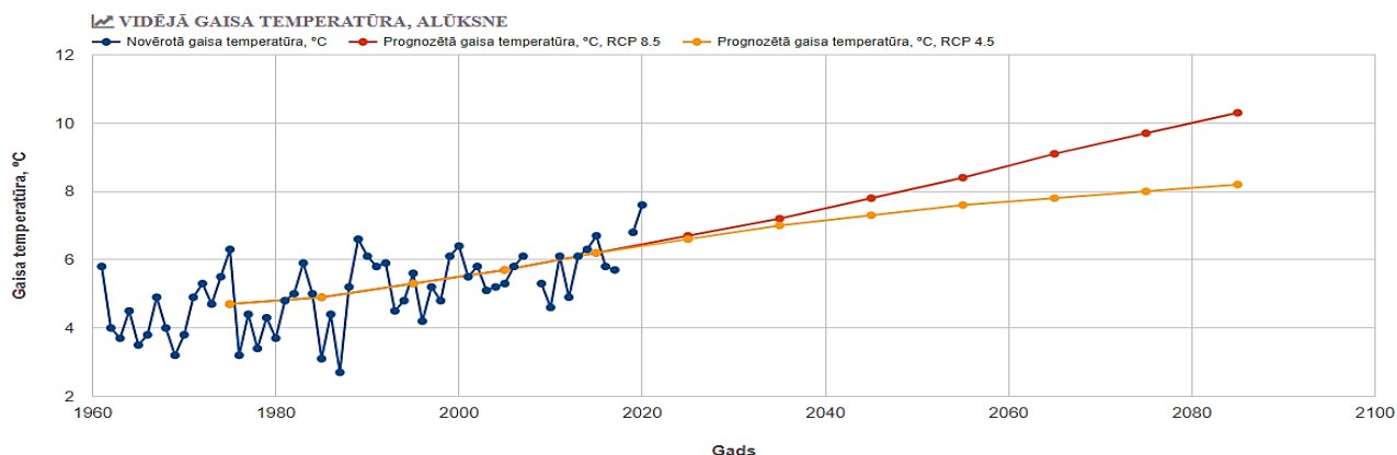
Attēls 10.1. Vidējā gaisa temperatūra Alūksnē, Avots LVĢMC
