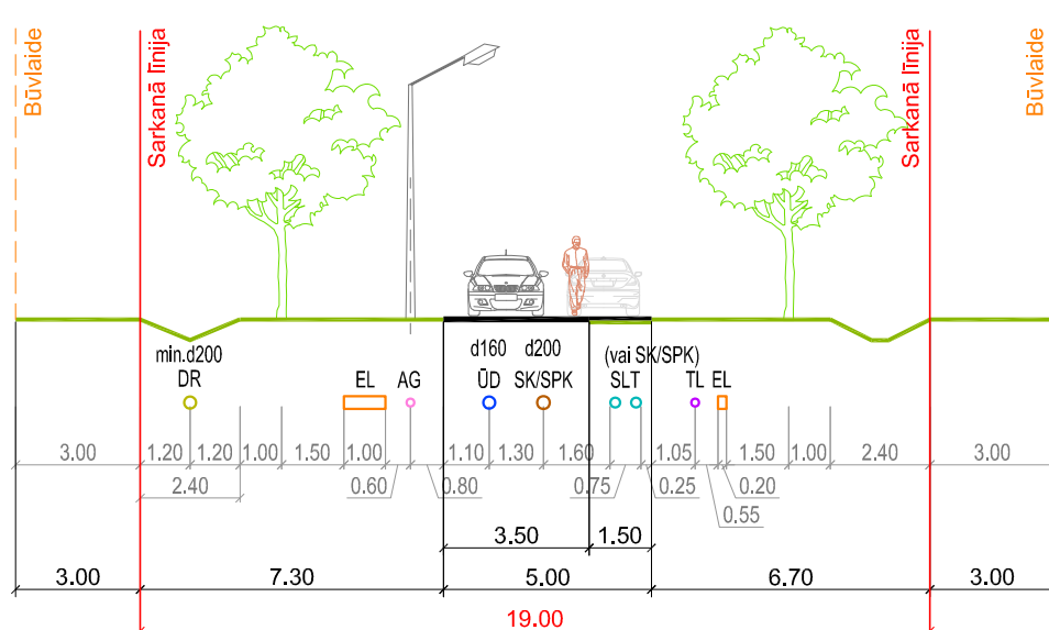
Šķēršprofils 2-2 Plānotā situācija
