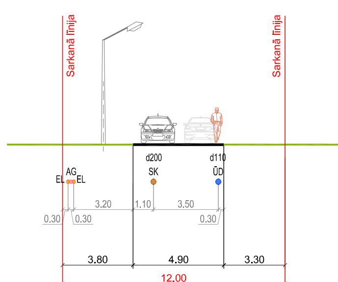
Šķēršprofils 12-12 Esošā / plānotā situācija
