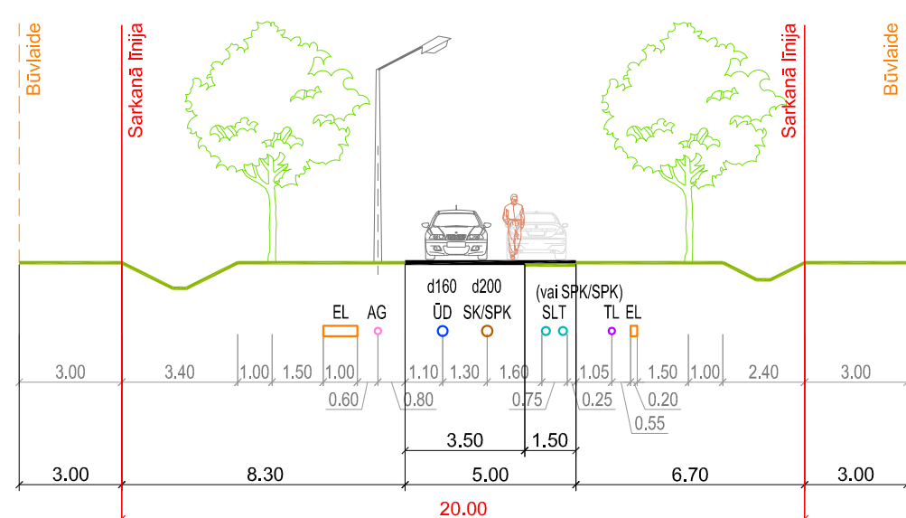
Šķēršprofils 1-1 Plānotā situācija
