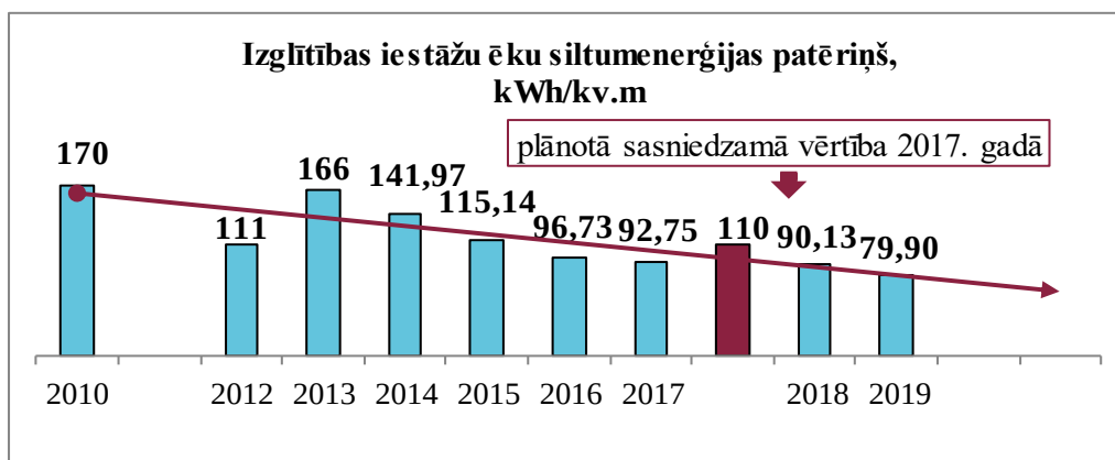
71. attēls. Izglītības iestāžu ēku siltumenerģijas patēriņa salīdzinājums
